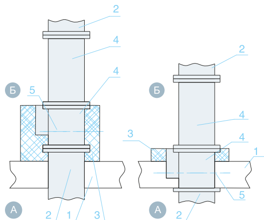
Схема установки в перекрытиях
