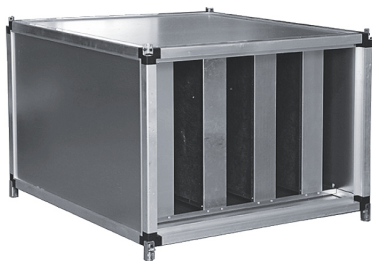
Шумоглушитель SHP
